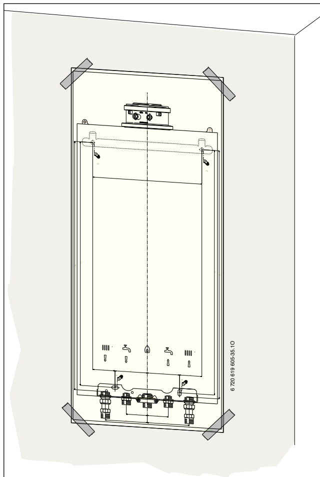
Рис. 9 Монтажный шаблон
