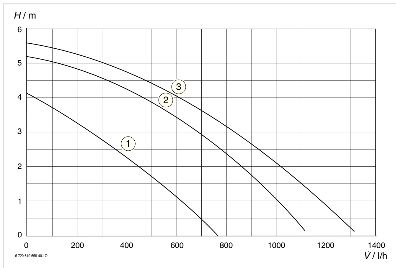
Рис. 34 Диаграмма насоса
