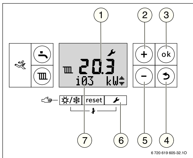
Рис. 35 Элементы управления
