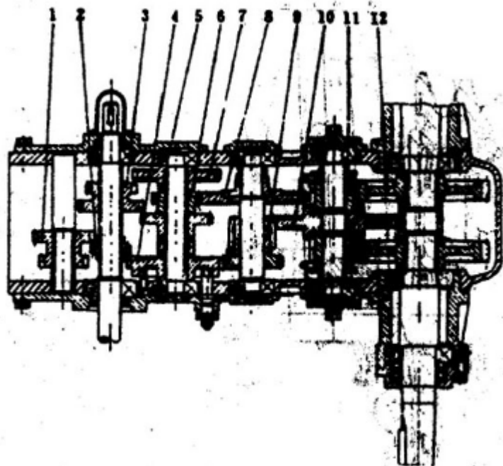
Рис. 4 Коробка передач
