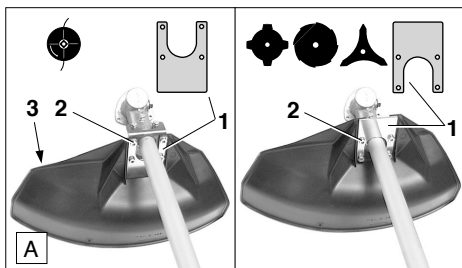
Монтажное положение А Монтажное положение В
