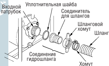
Рисунок 7. Подключение шлангов.
