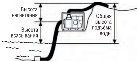
Рисунок 9. Установка мотопомпы.
