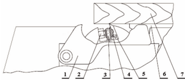
Рис.3. Регулировка ножей
