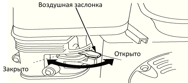
Воздушная заслонка
