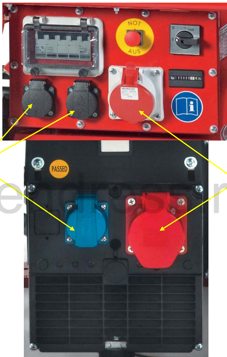
Рис. 4.4: Подключение потребителей
