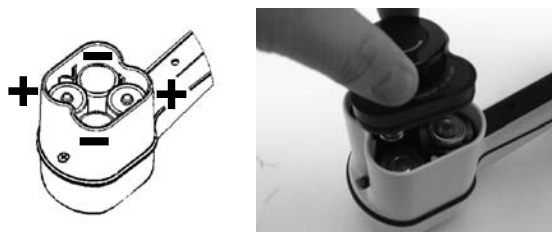
Рис. 2: Отсек батарей
