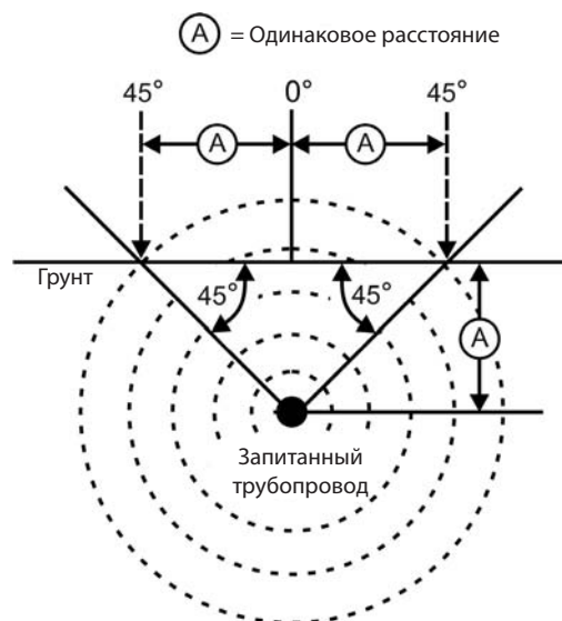
Рис. 22: Проверка искажения
