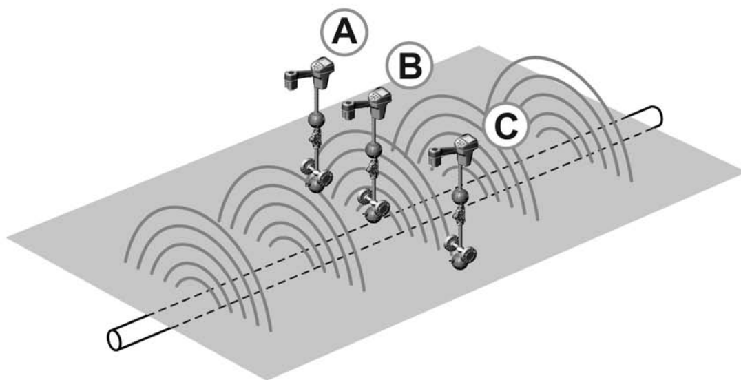
Рис. 23: Показания на дисплее в различных местоположениях прибора SR-20 (при обнаружении трассы магистрали)
