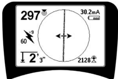
Рис. 24: 60 я Гц – частота пассивного обнаружения трассы магистрали
