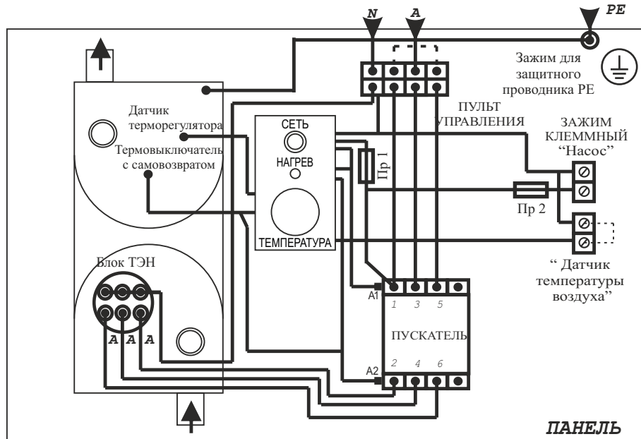
Рисунок 5. Электрическая схема подключения
