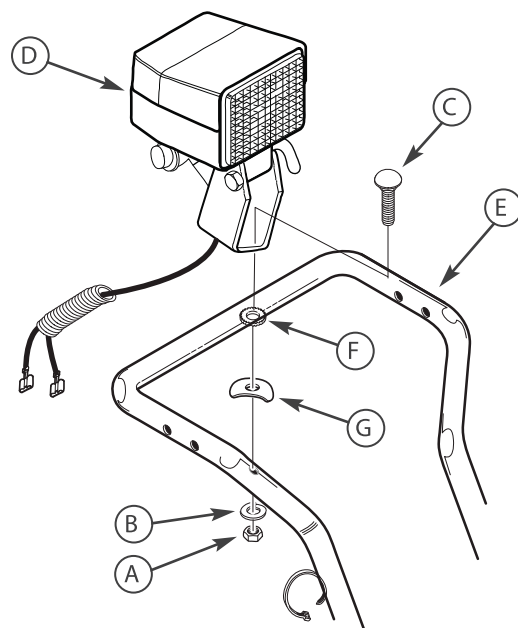
Сборка фары
