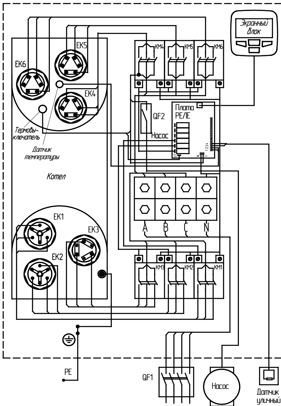
Рисунок 10. Схема подключения ЭВАH UNIVERSAL -72, 90
