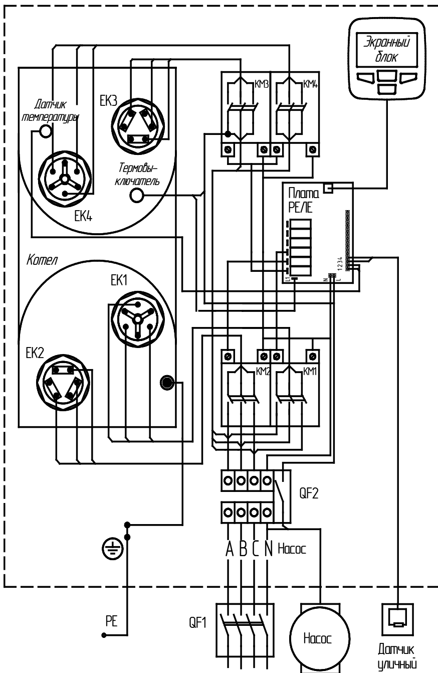
Рисунок 6. Схема подключения ЗВАН UNIVERSAL -42 - 12 -
