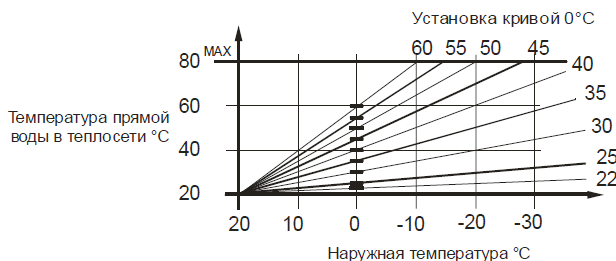
ОТОПИТЕЛЬНАЯ КРИВАЯ электрокотла, в которой по вертикальной шкале температура прямой воды по горизонтальной шкале температура наружного воздуха.
