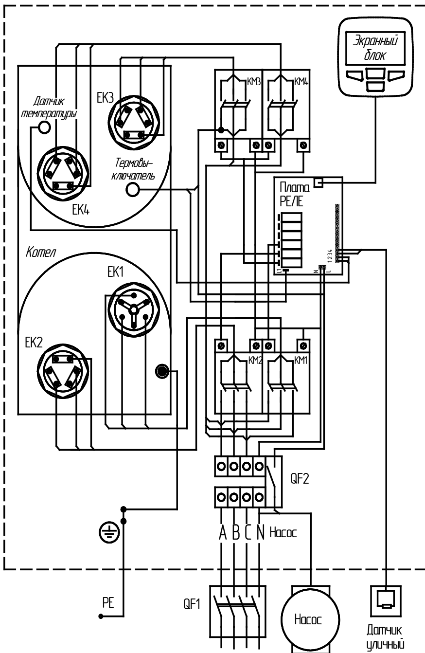
Рисунок 7. Схема подключения ЭВАН UNIVERSAL -48, 54 - 13 -
