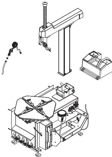
Рисунок 3 – Монтаж стойки шиномонтажного стенда
