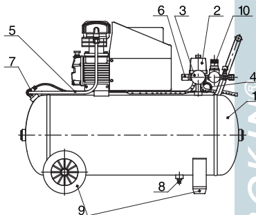
Рисунок 1 – Общее устройство компрессора с прямой передачей
