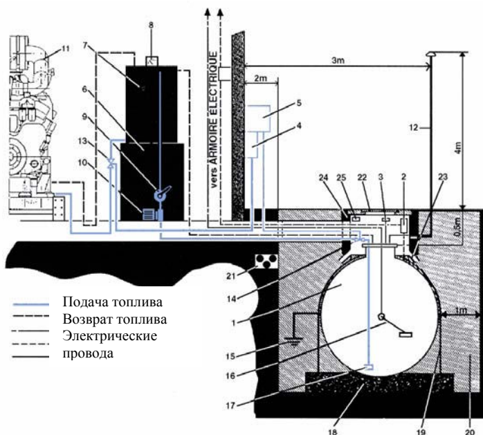
Рисунок 2.11: Пример установки
