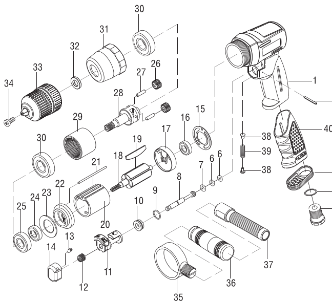
Рисунок 1 - Деталировка
