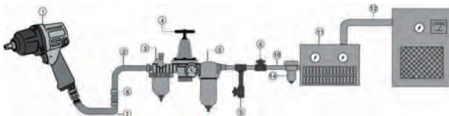
Рисунок 5 – Пневматическая схема подключения
