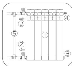
боковое (однотрубная система отопления)
