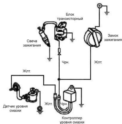
Схема управления двигателем с электрическим стартером
