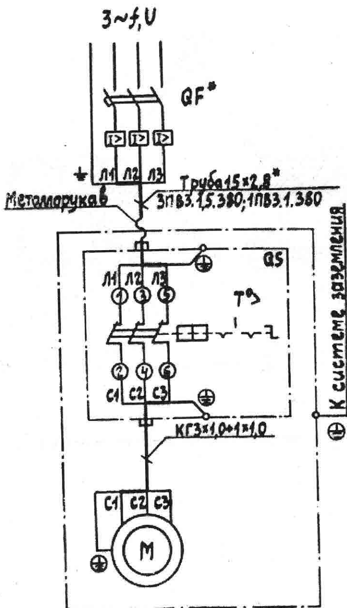
Рис. 39. Схема электрическая принципиальная и соединений установки компрессорной КВ-15
