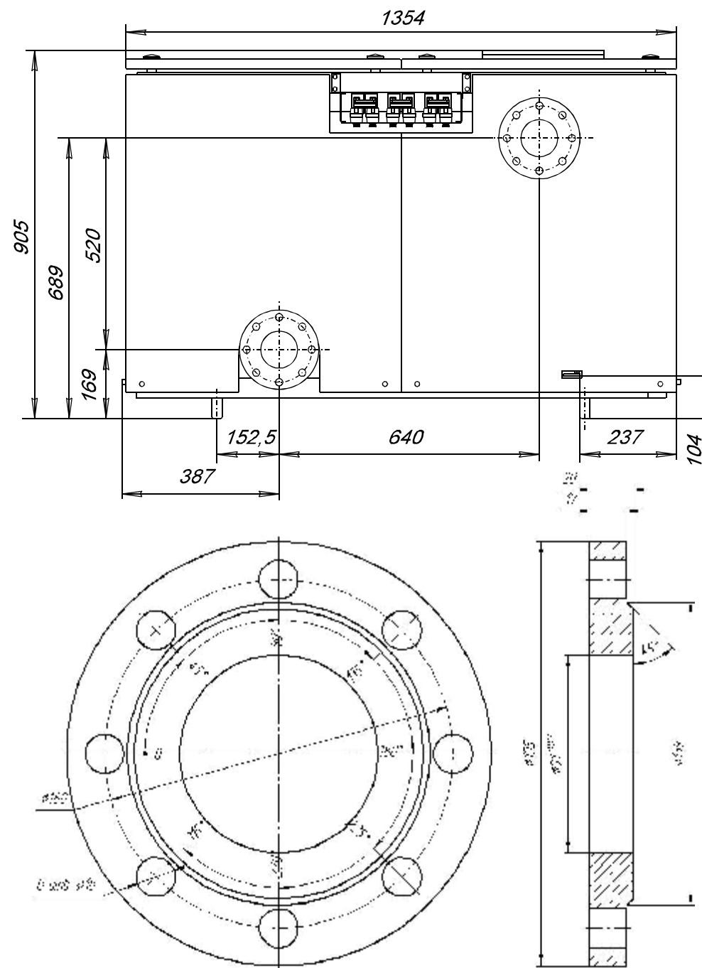
Рис. 4 Вид сзади
