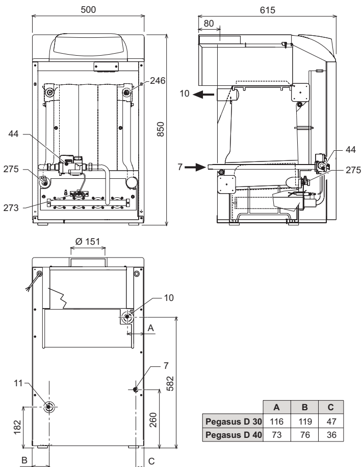
мал. 23 - Розміри і приєднувальні розміри мод. PEGASUS D 32 - 45
