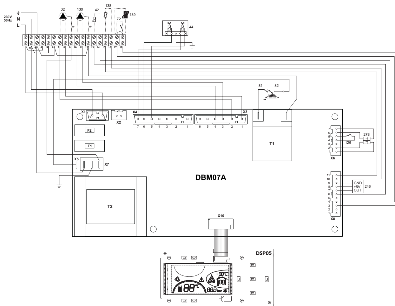
рис. 25 - Электрическая схема
