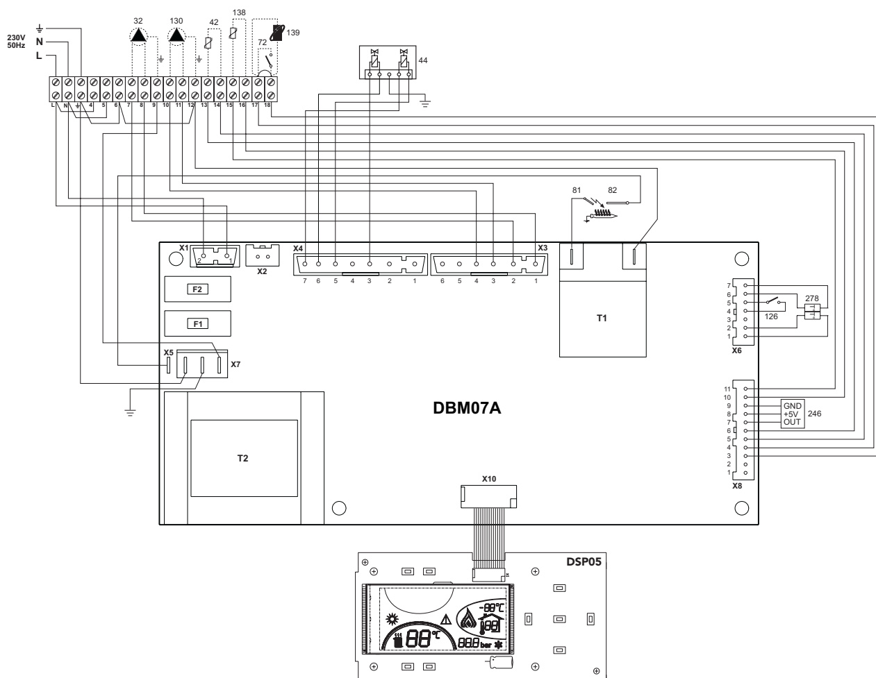
мал. 25 - Електрична схема
