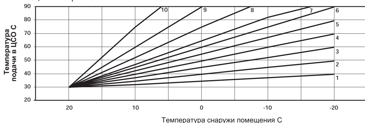
Компенсационные кривые
