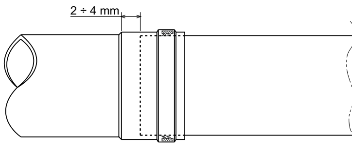
рис. 14 - Тепловое расширение
