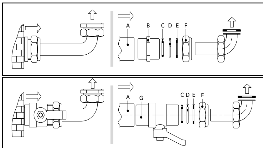
рис. 12 - Соединительный комплект
