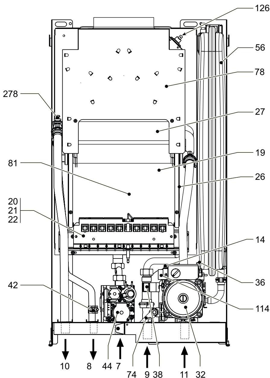
рис. 18 - Общий вид
