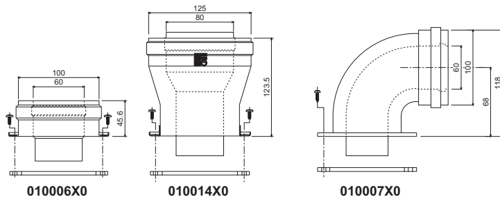
fig. 22 - Accessoires de départ pour conduits coaxiaux
