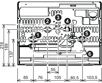
fig. 17 - Conexiones hidráulicas
