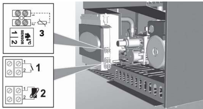
fig. 20 - Accesso alla morsettiera
