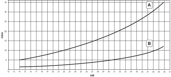
мал. 37 - Діафрагма тиску/потужність DIVAtop MICRO F 37 A GPL (зріджений нафтовий газ) B METAN
