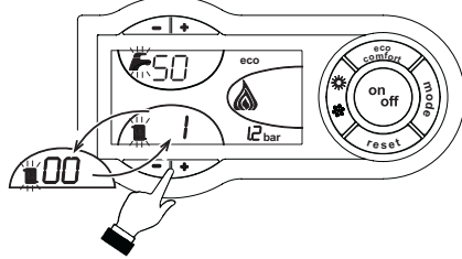
şek. 26 - TEST Modu (ısıtma gücü = %100)
