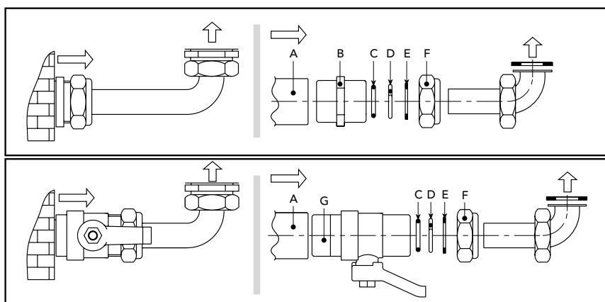
рис. 7 - Соединительный комплект
