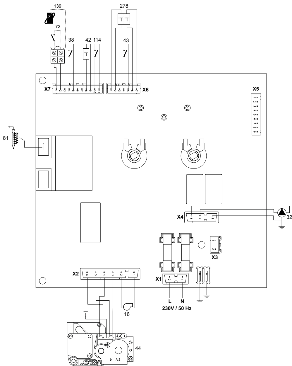
рис. 22 - Электрическая схема
