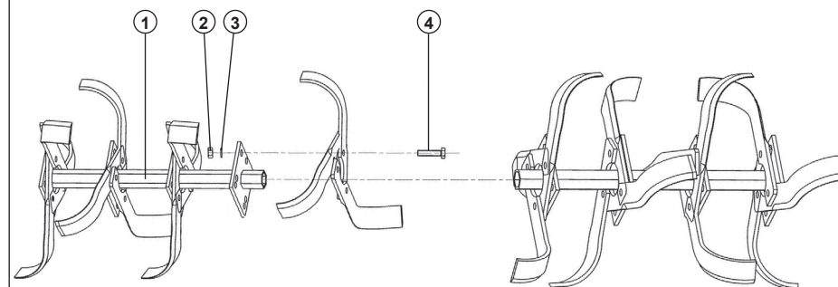
Схема сборки фрез
