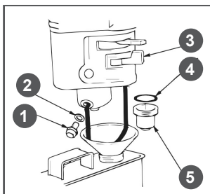
Рис. 25 Обслуживание фильтра-отстойника
