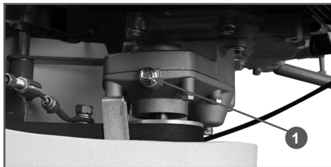
Рис. 11 Заправка масла в редуктор двигателя
