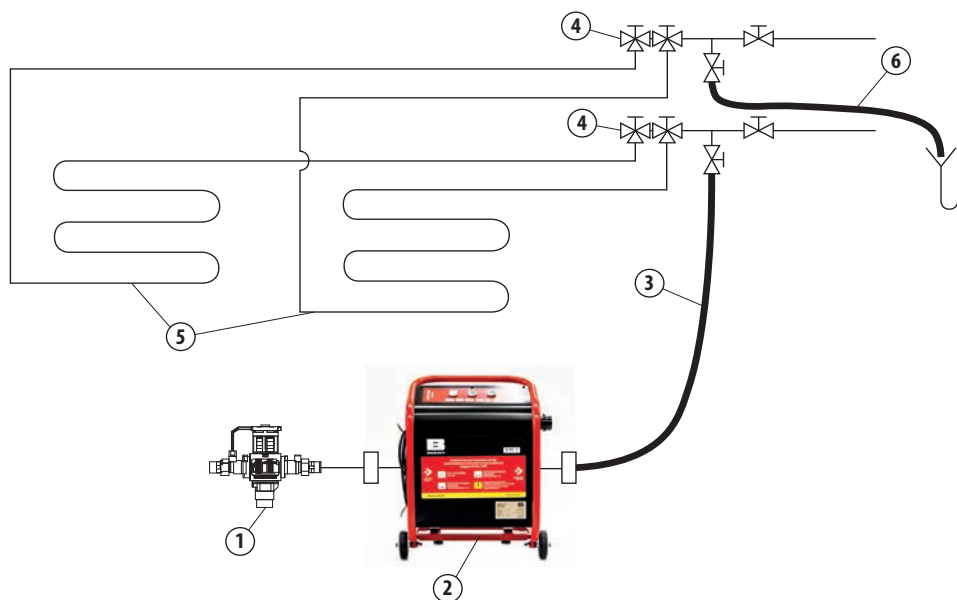
Схема подключения для промывки систем напольного отопления
