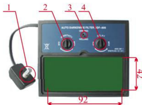
Рис.2 Светофильтр NWT II
