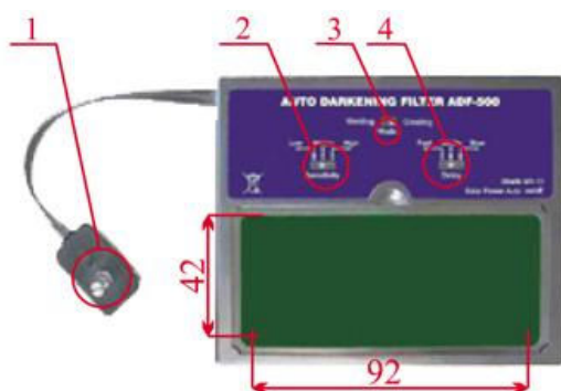
Рис.1 Светофильтр NWT
