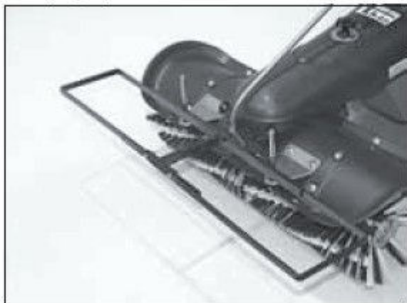
1) Наденьте раму на стержни.
