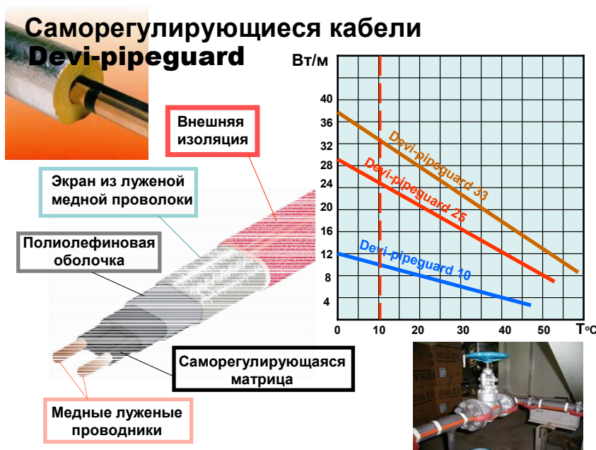
Рис. 3. Устройство саморегулирующегося нагревательного кабеля
