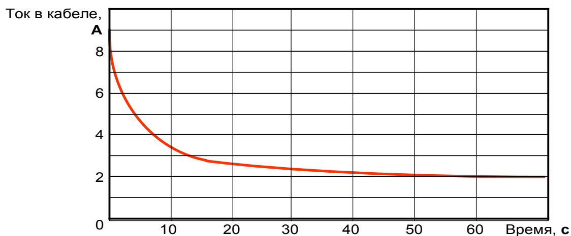
Рис.2. Пусковой ток саморегулирующегося кабеля при температуре -20°C.
