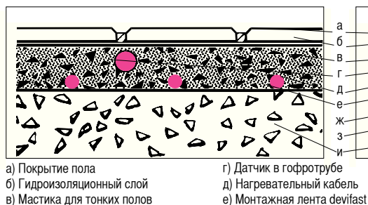
Рис.5. Тонкий пол на существующем бетонном полу.
