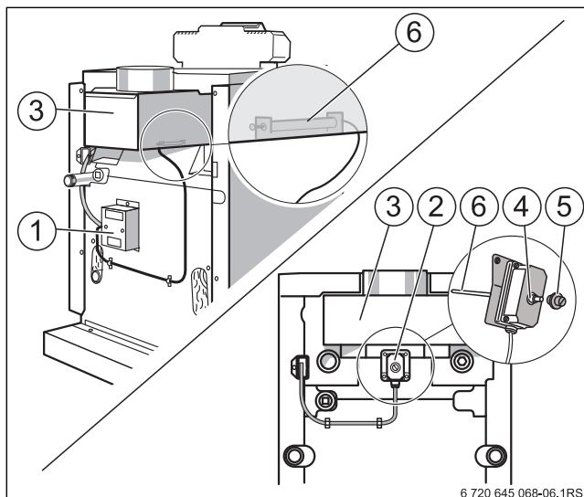
Рис. 10 Устройства контроля дымовых газов
