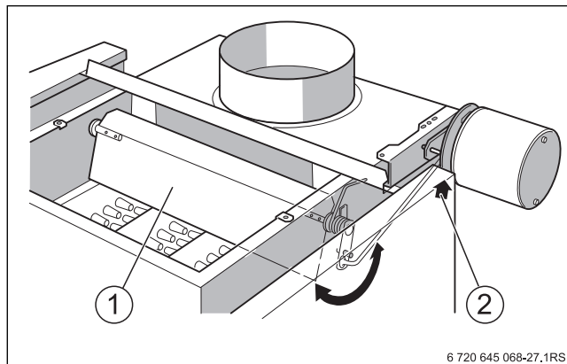
Рис. 38 Заслонка дымовых газов в положении "Закрыто"
