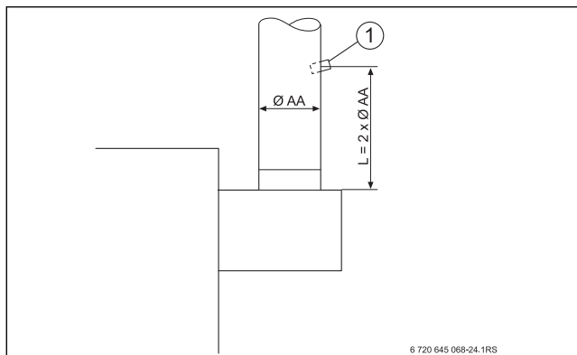
Рис. 34 Точка замера на дымовой трубе
