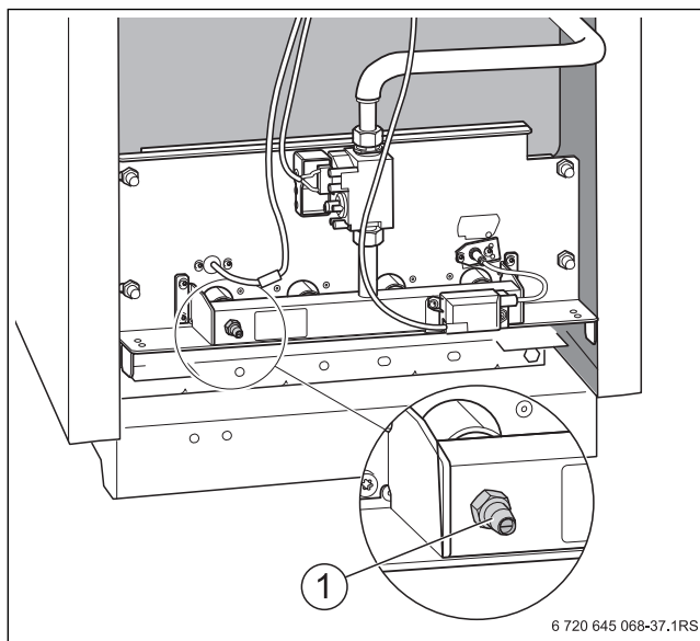
Рис. 45 Измерение давления на форсунках
