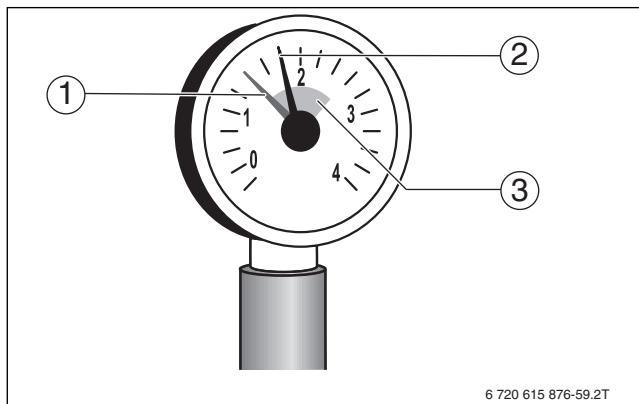
Рис. 44 Манометр для закрытых установок
