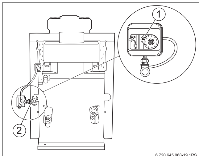
Рис. 8 Подключение газа
