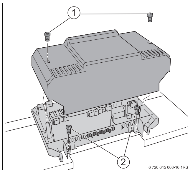
Рис. 15 Снятие верхней крышки
