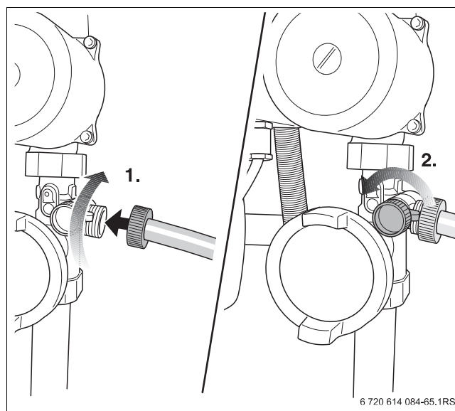
Рис 4 Подсоединение шланга
