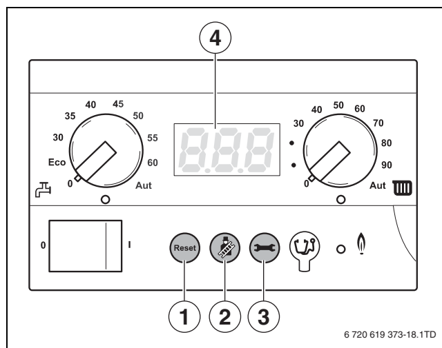
Рис 13 Пульт управления
