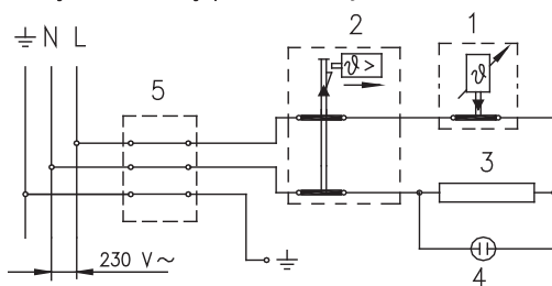
Schéma elektrického propojení
