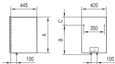
Прикључни и монтажни димензии на греалкаторот [mm]
