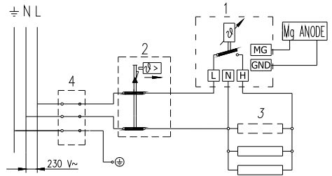
Das Schaltungsschema des Elektroanschlusses
