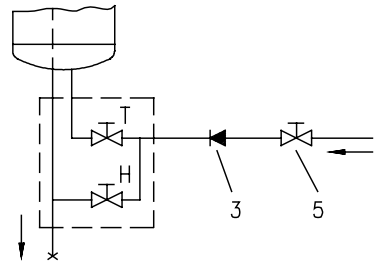
Das Durchflußsystem
