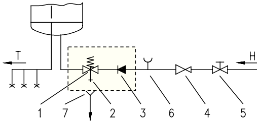
Das Drucksystem
