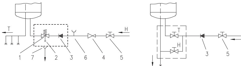
Uzavřený (tlakový) systém
