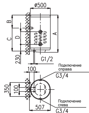
GBK 80 – 200
