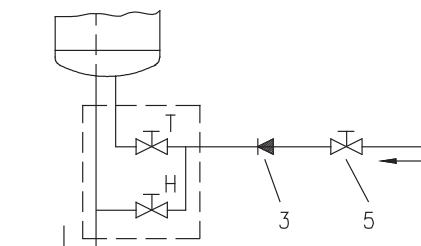
Avatud (loomuliku vooluga) süsteem
