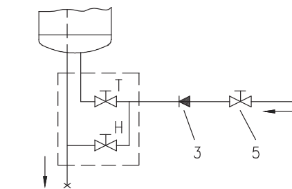
Отворен систем (преleven)
