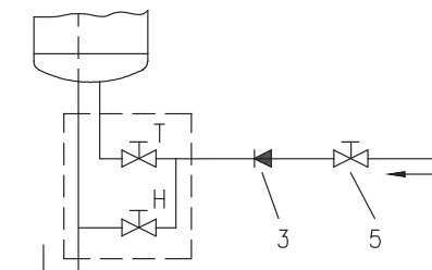
Odprti (netlačni) sistem
