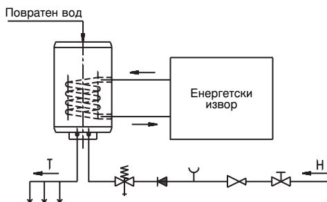
Отворен систем (преleven)
