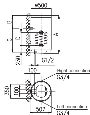
GBK 80 - 200
