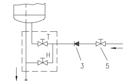
Otwarty system (nieciśnieniowy)
