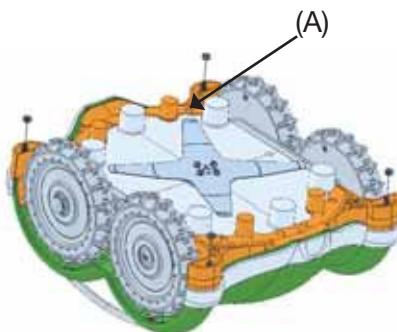
Отсоединение сенсоров края газона
