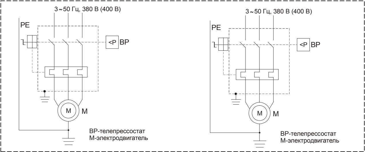
Рисунок 7 – Схема электрическая принципиальная для KP2095TB/500/11T
