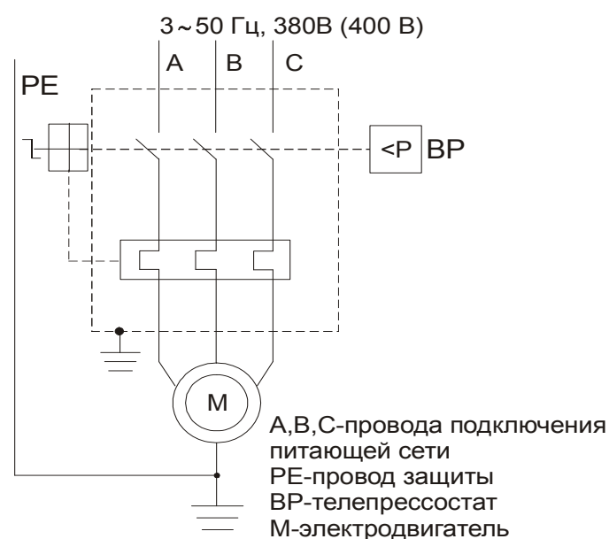
Рисунок 6 – Схема электрическая принципиальная для КР2095/100/5.5Т, КР2095/270/5.5Т, КР2095/270В/5.5Т, КР2095/500/5.5Т
