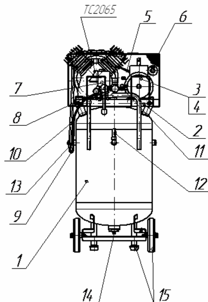
Рисунок 2 – Общий вид компрессора КР2065/100/2.2Т, КР2065/100/2.2
