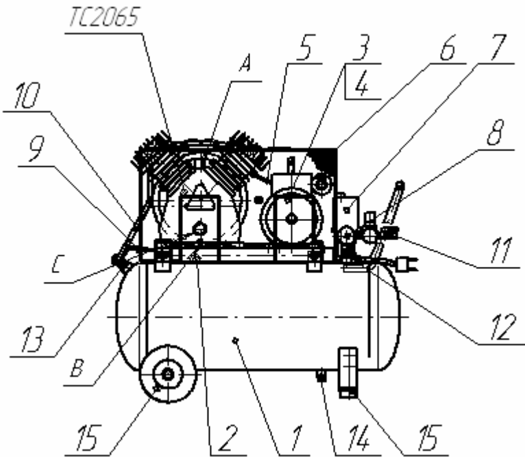
Рисунок 1 – Общий вид компрессора КР2065/50/2.2Т, КР2065/50/2.2
