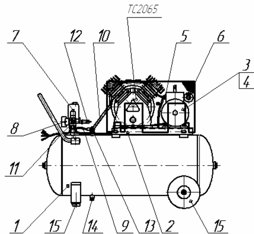
Рисунок 2 – Общий вид компрессора КР2065/100/2.2Т, КР2065/100/2.2
