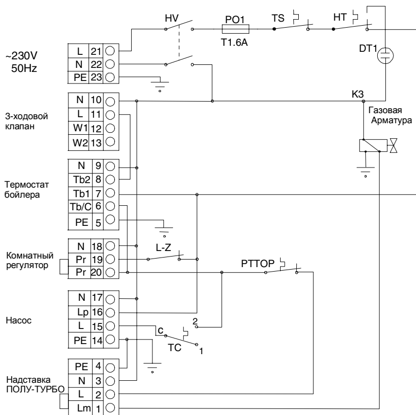
Рис. 5б – Схема электрического подключения котла 60 PLO
