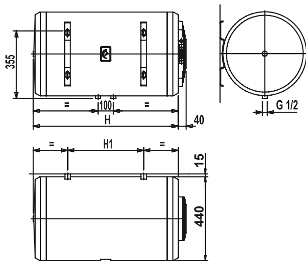
Горизонтальные модели
