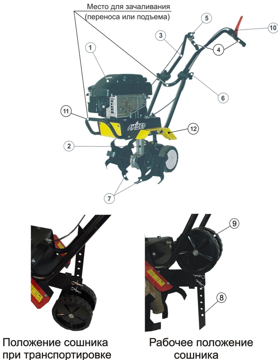
Рис. 1. Мотокультиватор
