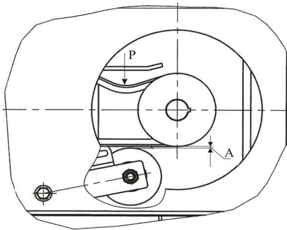
Рис. 5. Схема регулировки (вид с верху двигатель не показан)
