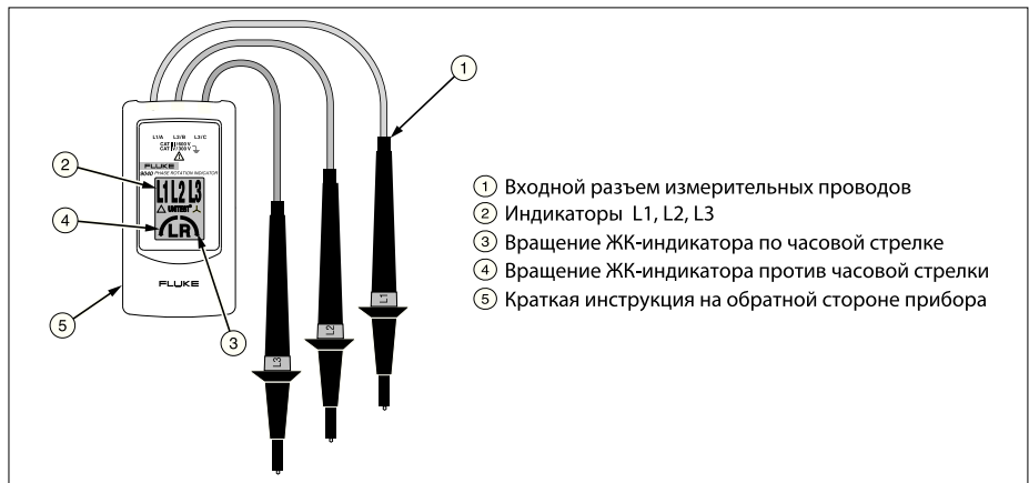
Рис. 1. Указатель порядка чередования фаз 9040
