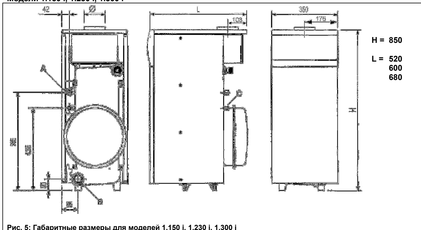
Рис. 5: Габаритные размеры для моделей 1.150 i, 1.230 i, 1.300 i
