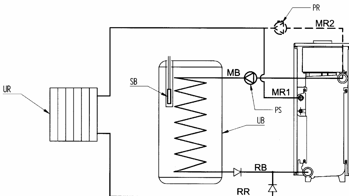
Рис. 11: Схема гидравлического присоединения бойлера
