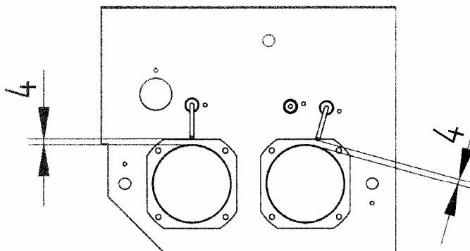
Рис. 21 Расположение электродов зажигания
