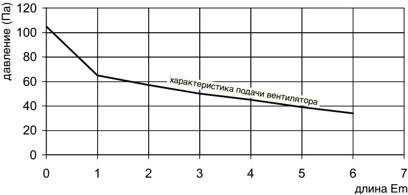
Подача вентилятора Ø 60/100 мм
