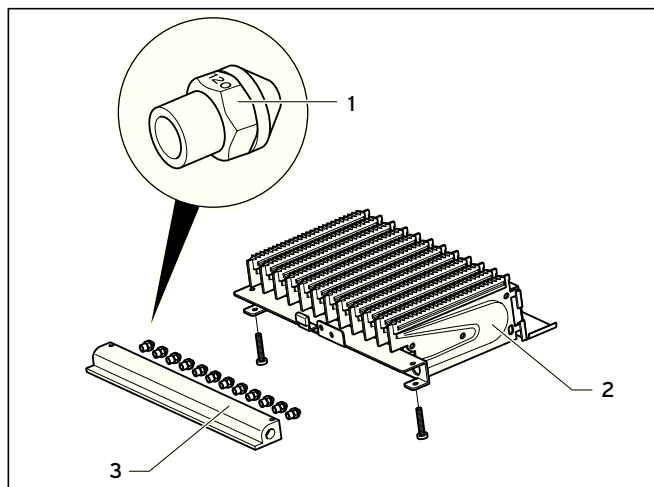
Рис. 6.6 Маркировка сопла
