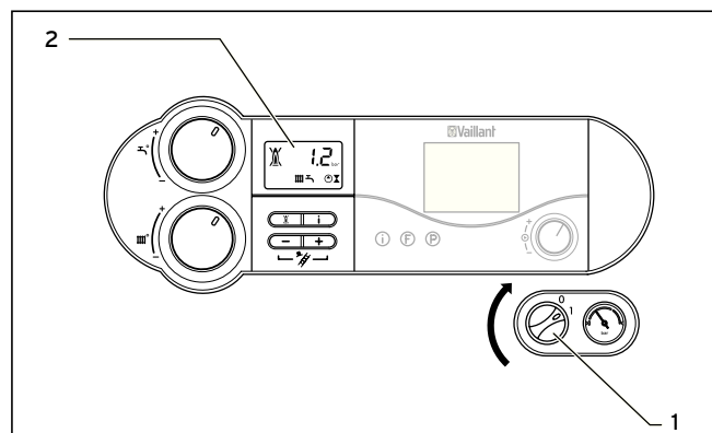
Мал. 4.6 Вмикання приладу (тут зображено: atmoTEC/turboTEC plus)
